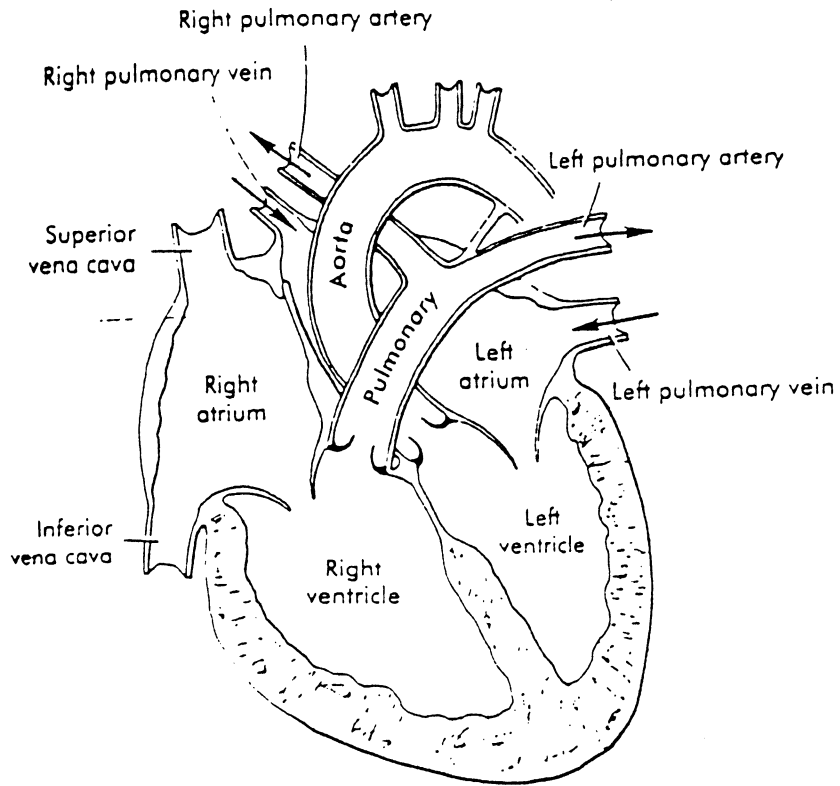
Normal heart
